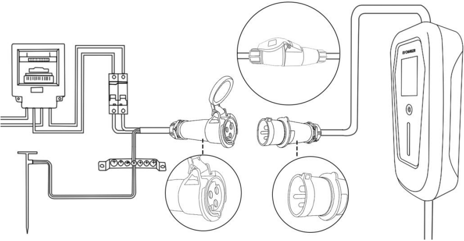
③ 单相电源 32A7KW 设备接线效果图
