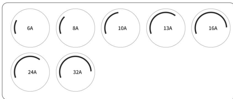
32A 规格型号随车充电电流调节档位示意图
