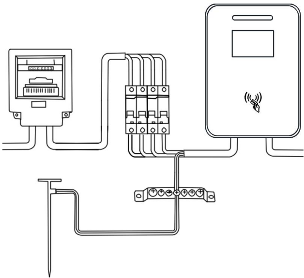
②三相电设备接线效果示意图
